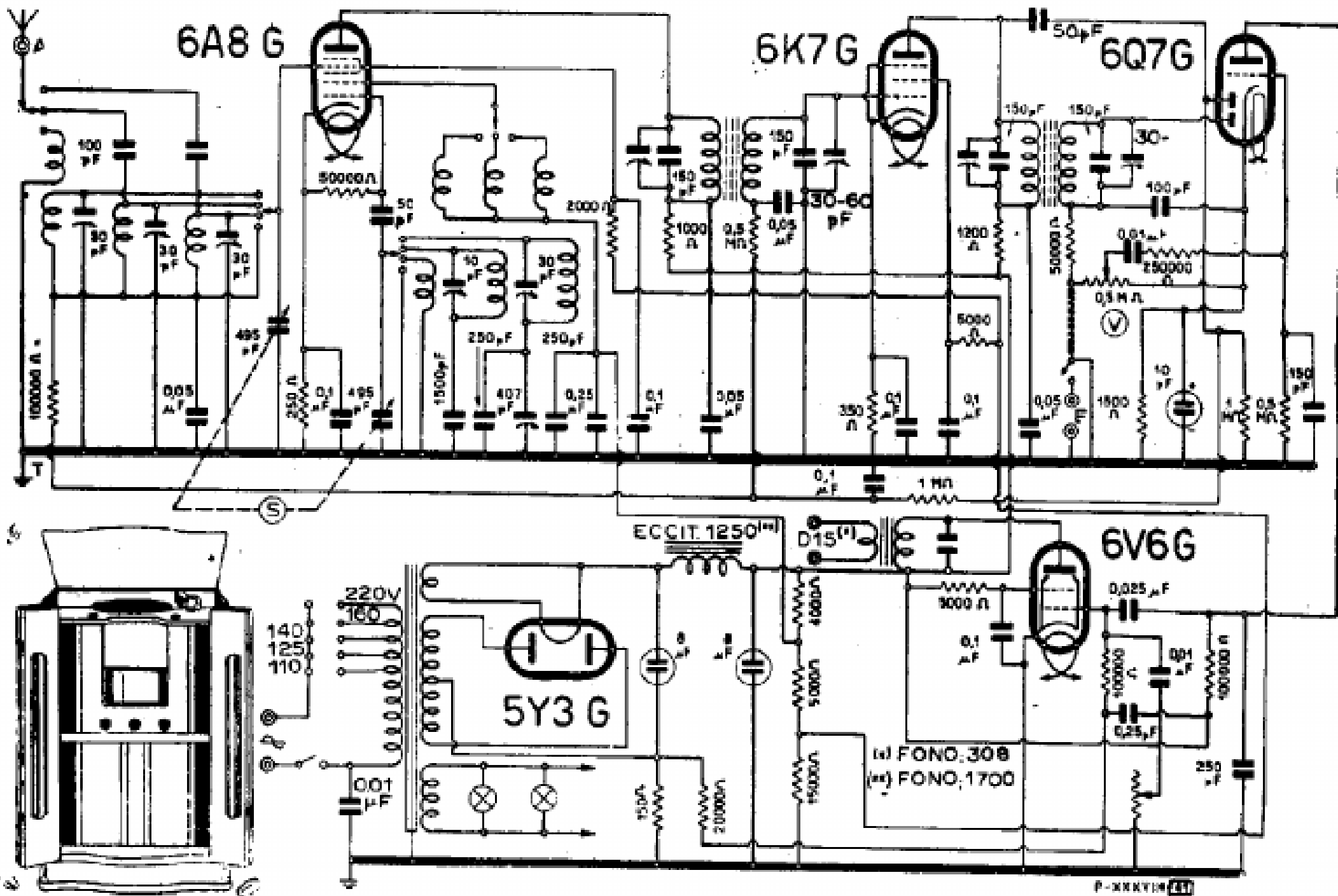
WATT RADIO - MOD. "FRECCIA"
